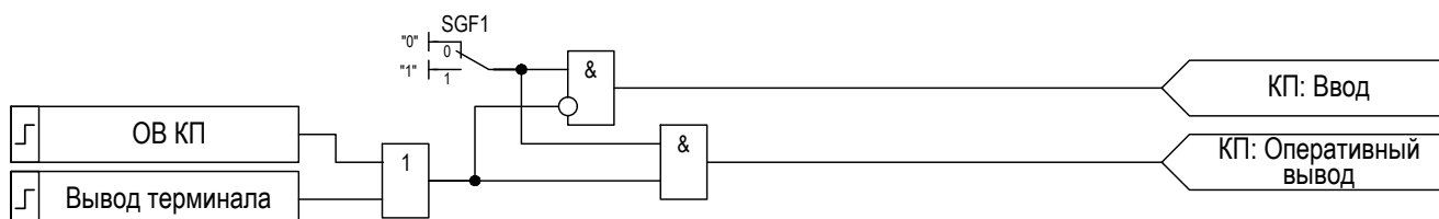
Рисунок 2.45 – Функциональная схема управления режимами работы функционального блока «КП»
